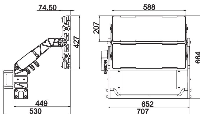
Montavimo padėties
