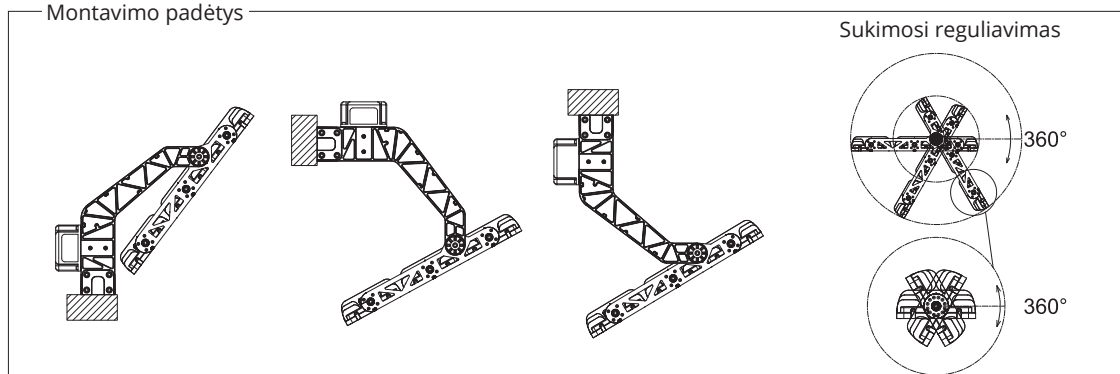
Montavimo padėties
